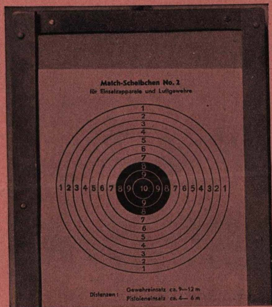
Schießkasten-Oberteil mit eingesteckter Scheibe. Der nicht sichtbare Unterfteil enthält die Figuren-Drehvorrichtung.
