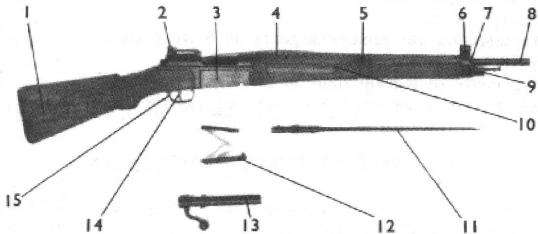
Fig. 1. — Fusil de 7,5 mm modèle 1936 (démonté).
