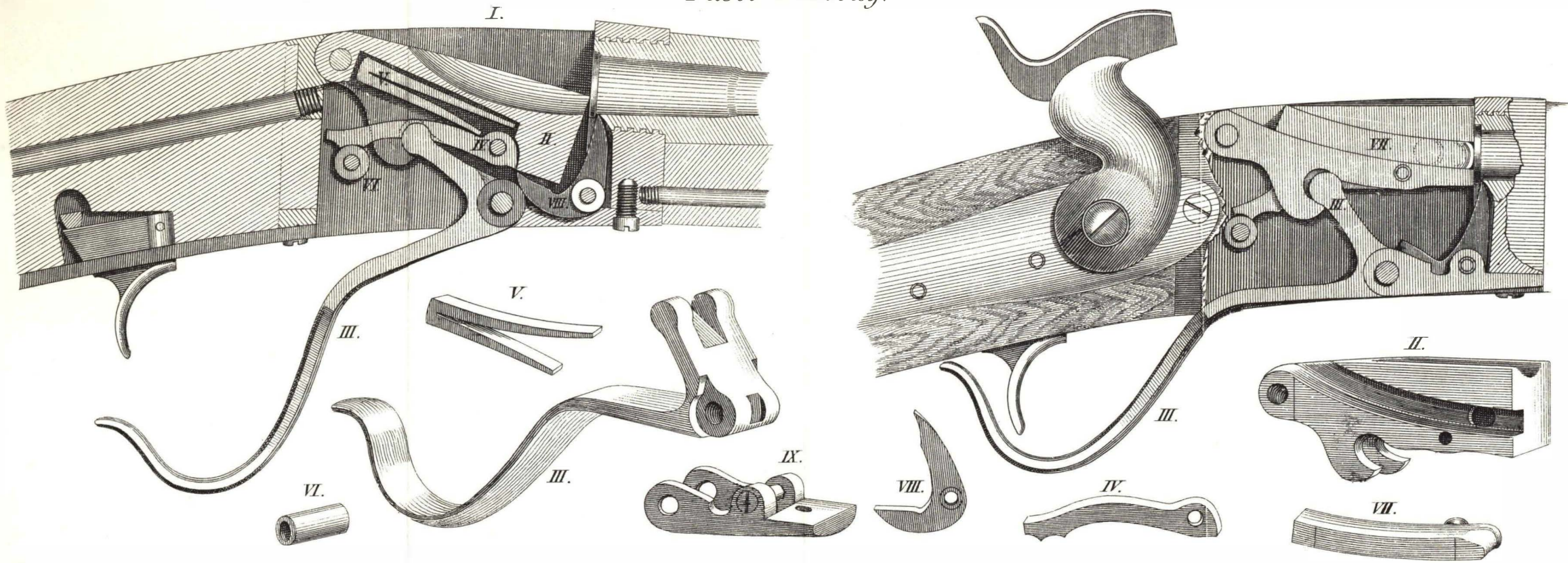
I. Verschlusskasten. I. Boîte de culasse.
