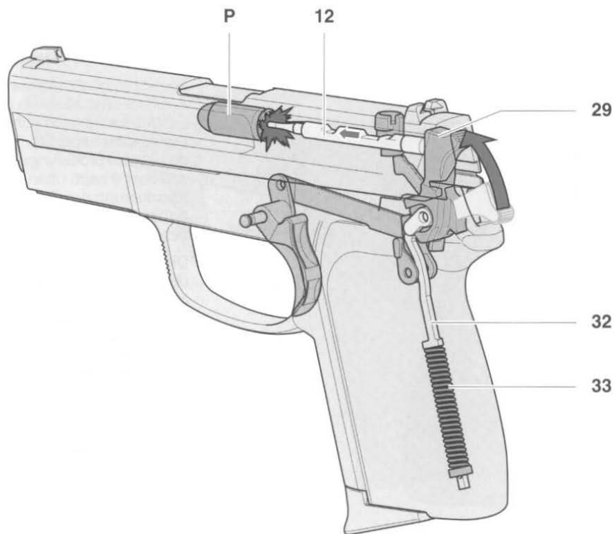
Abb. 21, Geschoss wird abgefeuert
