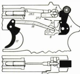
Abb. 2. - Innere Sicherung. Ruhestellung bei entschärfter Pistole
