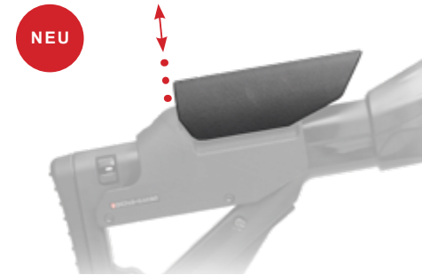
Art. Nr. 14.9747.01-14.9747.10 G+E Stgw 90 Zusatzerhöhung Schiebekolben Größen (Höhen): 2.5/5/7.5/10/12.5/15/17.5/ 20/22.5 und 25mm
