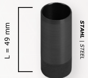
Schutzkappe, gerändelt Ø 20 mm Protection cap, curled Ø 20 mm (M18x1)
