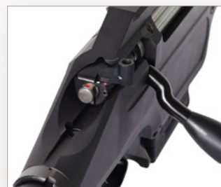
3-Stellungs Schlagbolzensicherung 3-position firing pin safety
