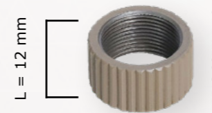
Mündungsschutz Ø 23 mm Protection cap Ø 23 mm (M18x1 left)
