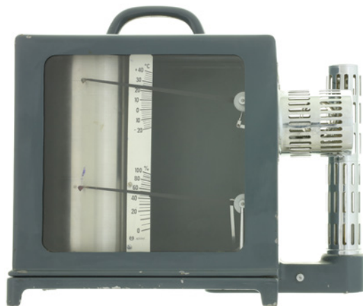
62923 CHF 60.- 284484 Thermo-Hygrograph Haenni KRK 508 mit mechanischem Uhrwerk. Mechanischer Daten-Thermo-Hygrograph KRK 508, Temperatur/Messbereich: -20 ..+40°C, Messgenauigkeit: ± 1°C. Relativer Feuchte/Messbereich: 0 .. 100%r.F. Messgenauigkeit: ± 4%r.F. Antrieb mechanisches Uhrwerk, aufziehbar mit Schlüssel. Registrierzeit umschaltbar: 24 Stunden / 175 Stunden (7 Tage). Gehäuse: grau lackiertes Metall mit Sichtfenster, Abmessungen 285 x 200 x 135 mm. 1 Aufziehschlüssel, Schlüssel für die Vorderseite fehlt, aber Schloss ist offen. Zustand 1
