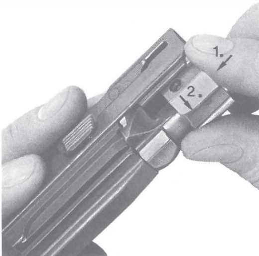
Verschlusskopf ausbauen
