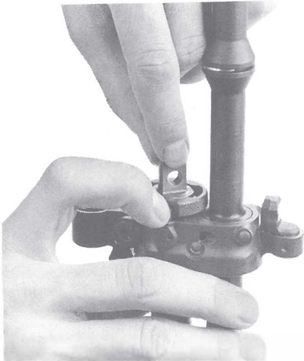
Gasdüse ausbauen
