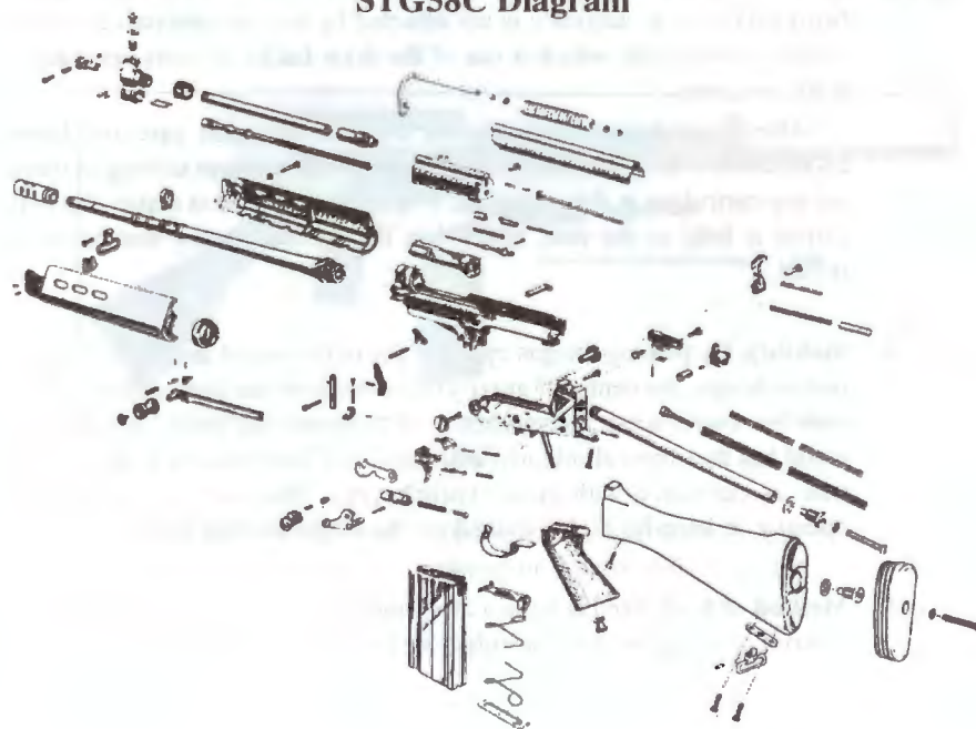
STG58C Diagram
